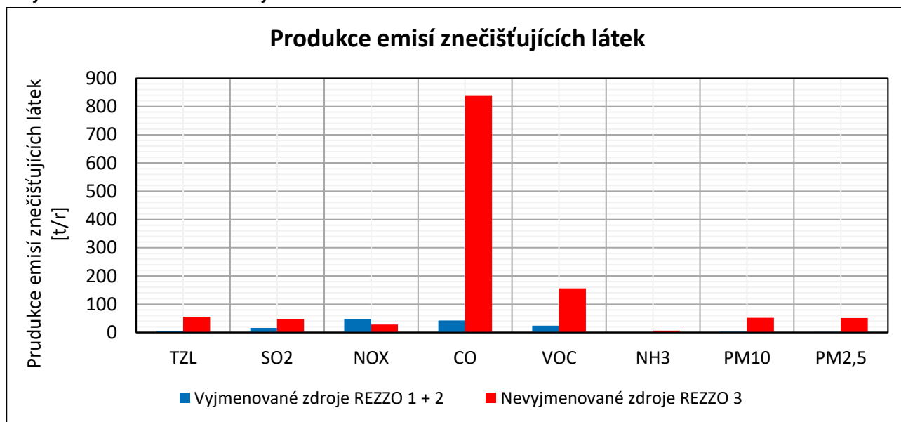
Graf C-4: Produkce emisí znečišťujících látek
