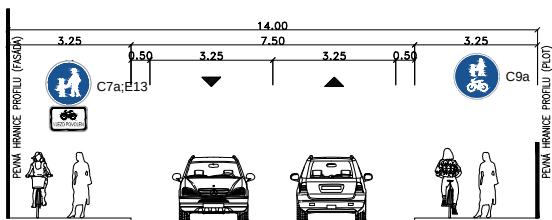
ŘEZ 8B _ Děčín - Ústecká (varianta se stezkami pro pěší a cyklisty)
