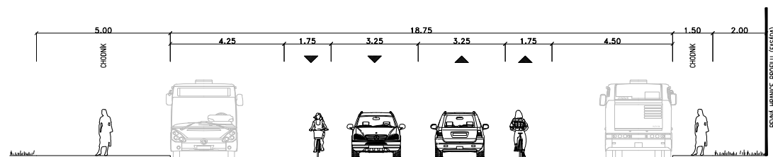
ŘEZ 3A _ Děčín - Československé mládeže (s cyklopruhu)
