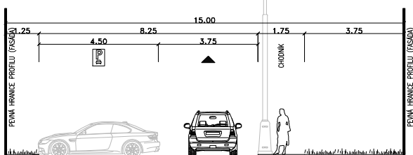
ŘEZ 4 _ Děčín - Práche (STAV)
