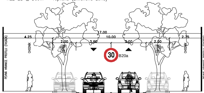
ŘEZ 2B _ Děčín – Teplická (zklidňená zóna)
