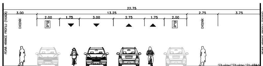
ŘEZ 14A _ Děčín - 28. října (cyklopruhy)
