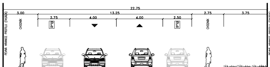
ŘEZ 14 _ Děčín - 28. října (STAV)
