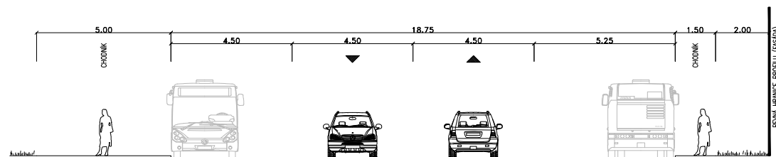
ŘEZ 3 _ Děčín - Československé mládeže (STAV)
