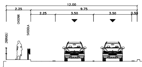
ŘEZ 7 _ Děčín – "Nový most" (STAV)
