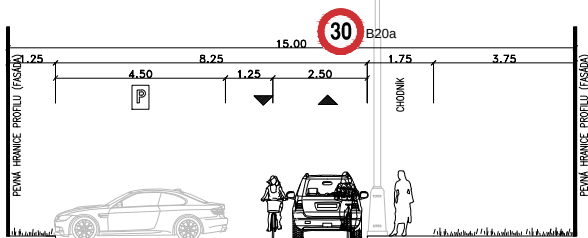
ŘEZ 4A _ Děčín - Práche (cykloobousměrka s cyklopiktokoridorem)
