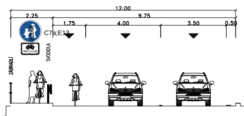
ŘEZ 7A _ Děčín – "Nový most" (varianta s cyklopruhy a povoleným vjezdem kol na chodník)
